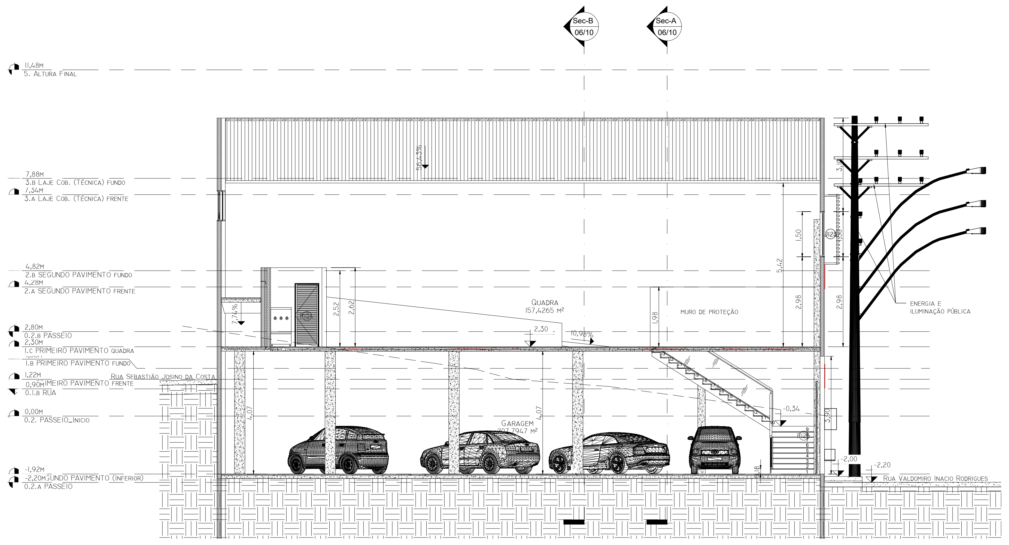
1 CORTE TRANSVERSAL "E" 1 : 75
