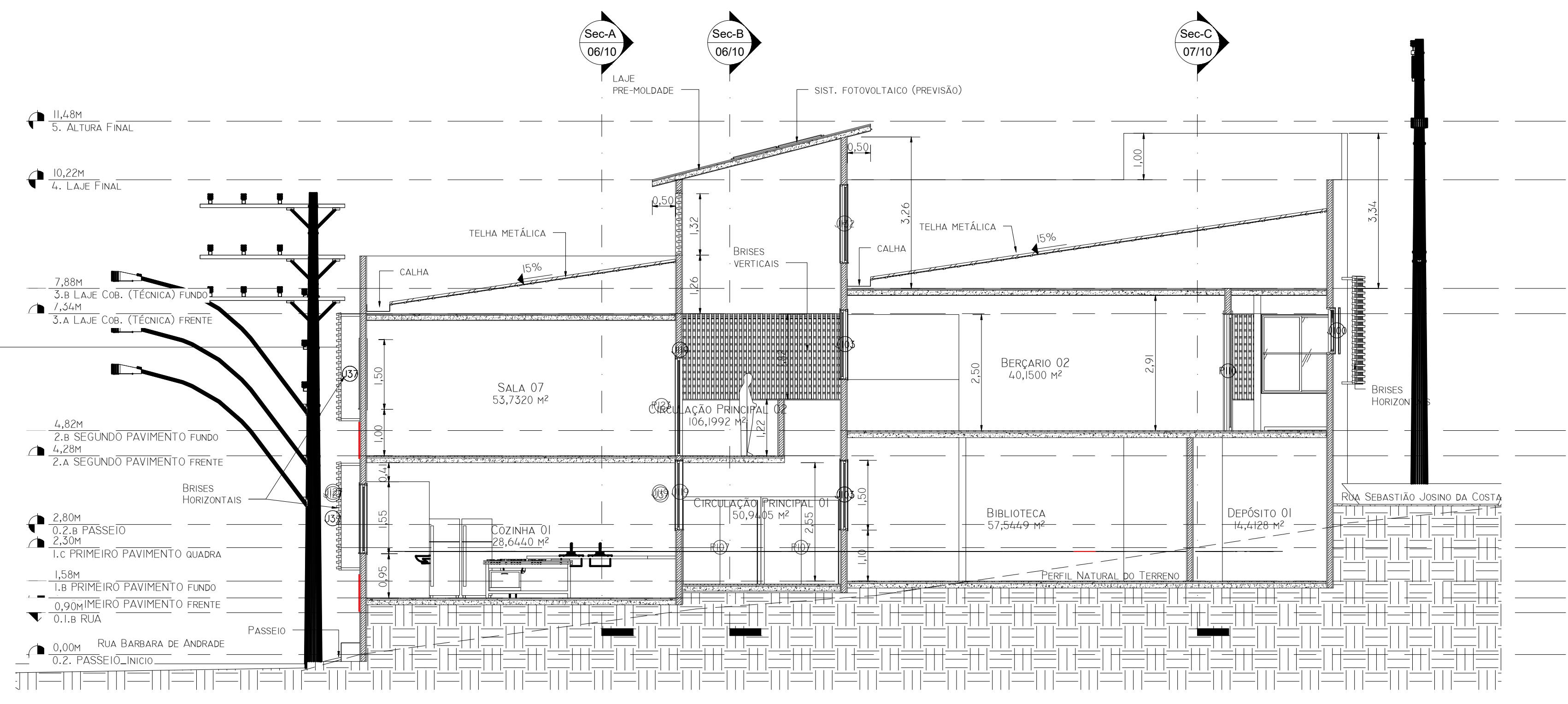
2 CORTE TRANSVERSAL "G" 1 : 75
