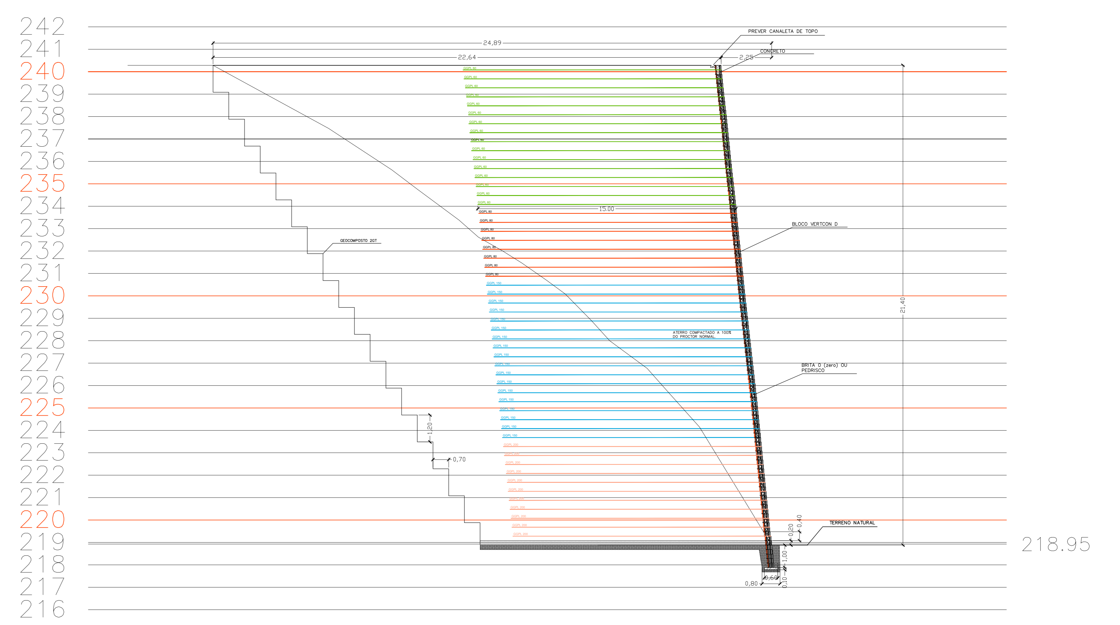
SEÇÃO 04 TRANSVERSAL DO MURO VERTCON D - H MAX. = 21,40m ESCALA: 1:100
