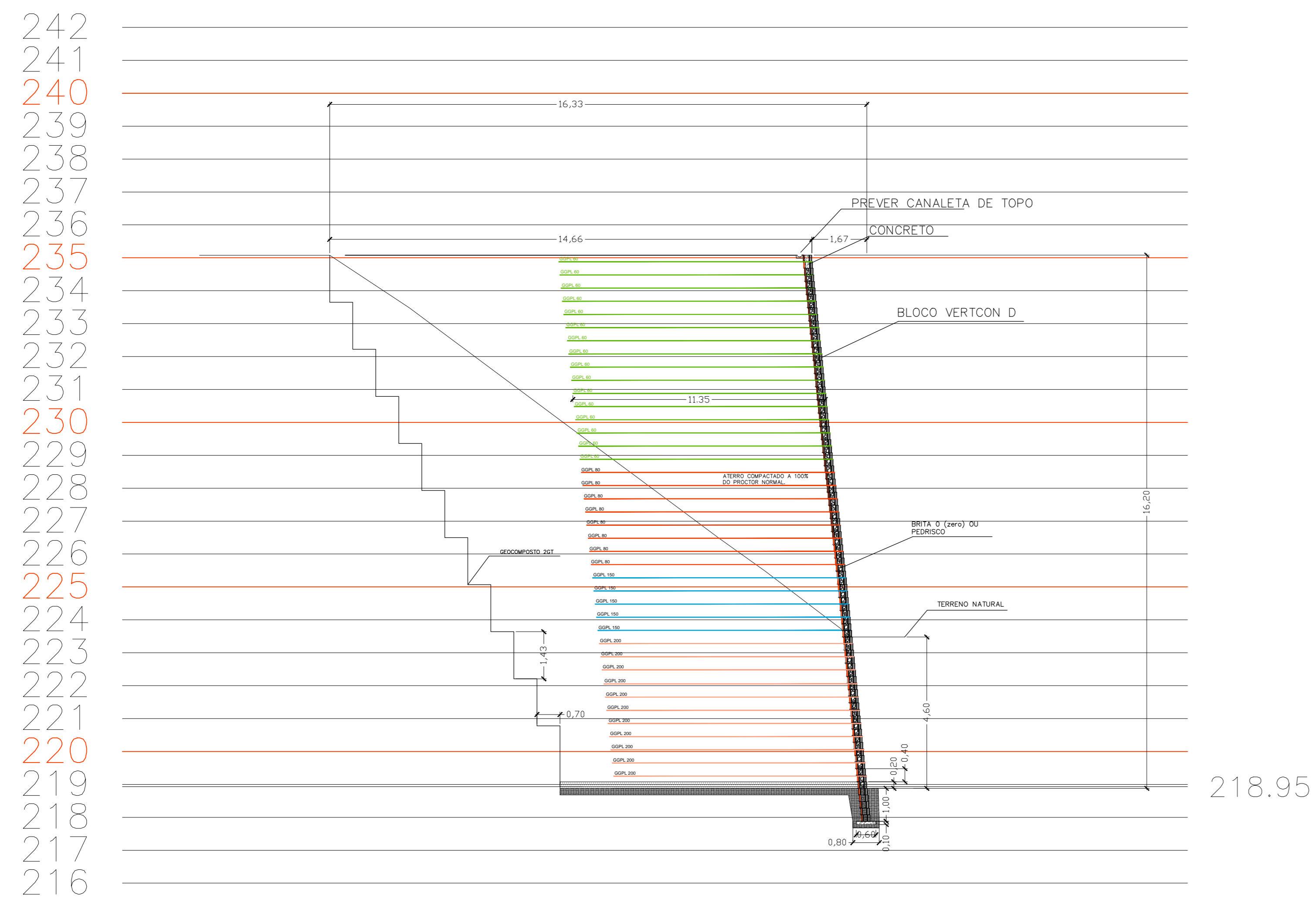
SEÇÃO 01 TRANSVERSAL DO MURO VERTCON D - H MAX. = 16,20m ESCALA: 1:100
