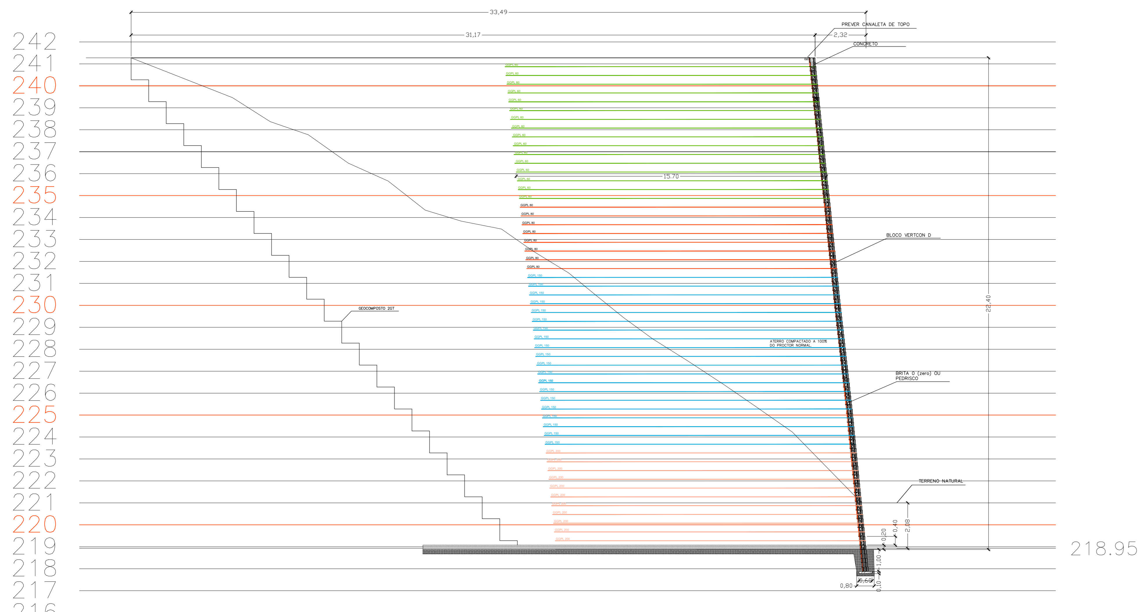
SEÇÃO 03 TRANSVERSAL DO MURO VERTCON D - H MAX. = 22,40m ESCALA: 1:100
