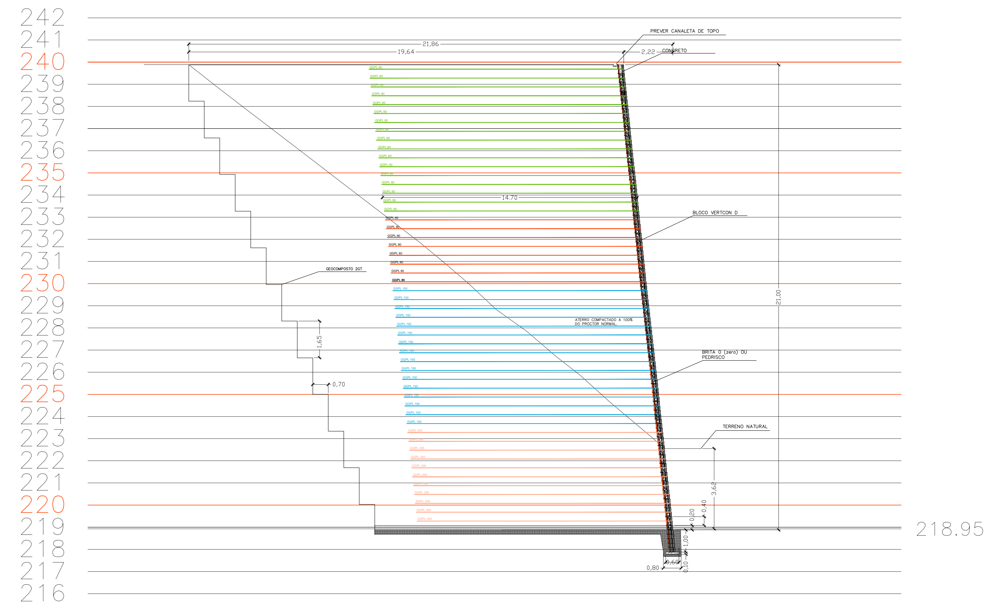
SEÇÃO 02 TRANSVERSAL DO MURO VERTCON D - H MAX. = 21,00m ESCALA: 1:100
