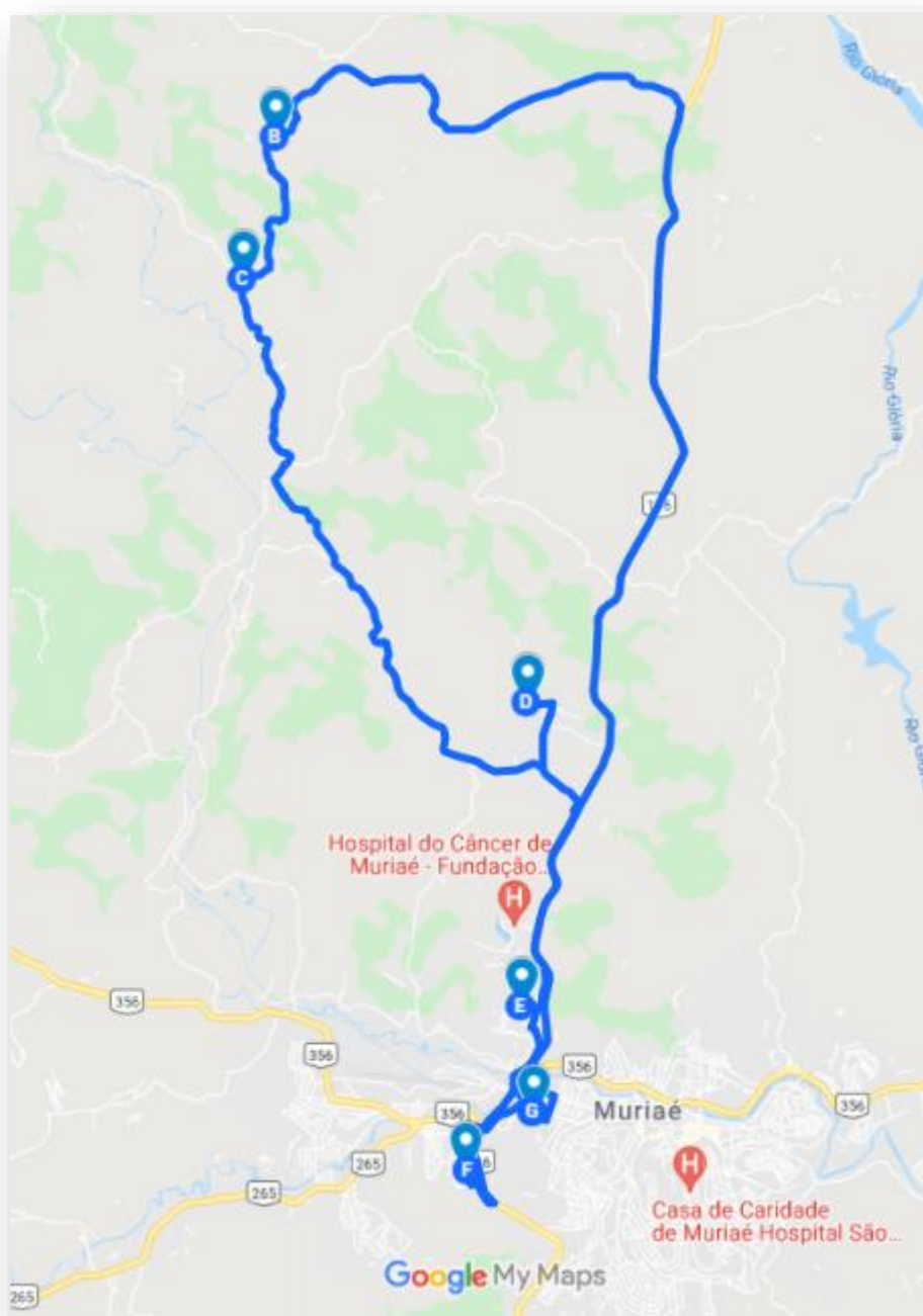
Imagem 1: Projeto Básico da linha Capetinga/Muriaé
