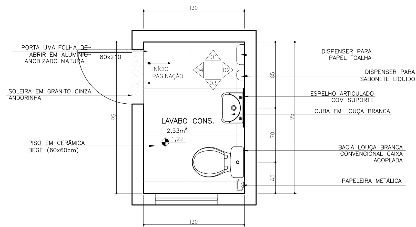
PLANTA LAYOUT LAVABO 01-Primeiro pavimento ESCALA 1:25
