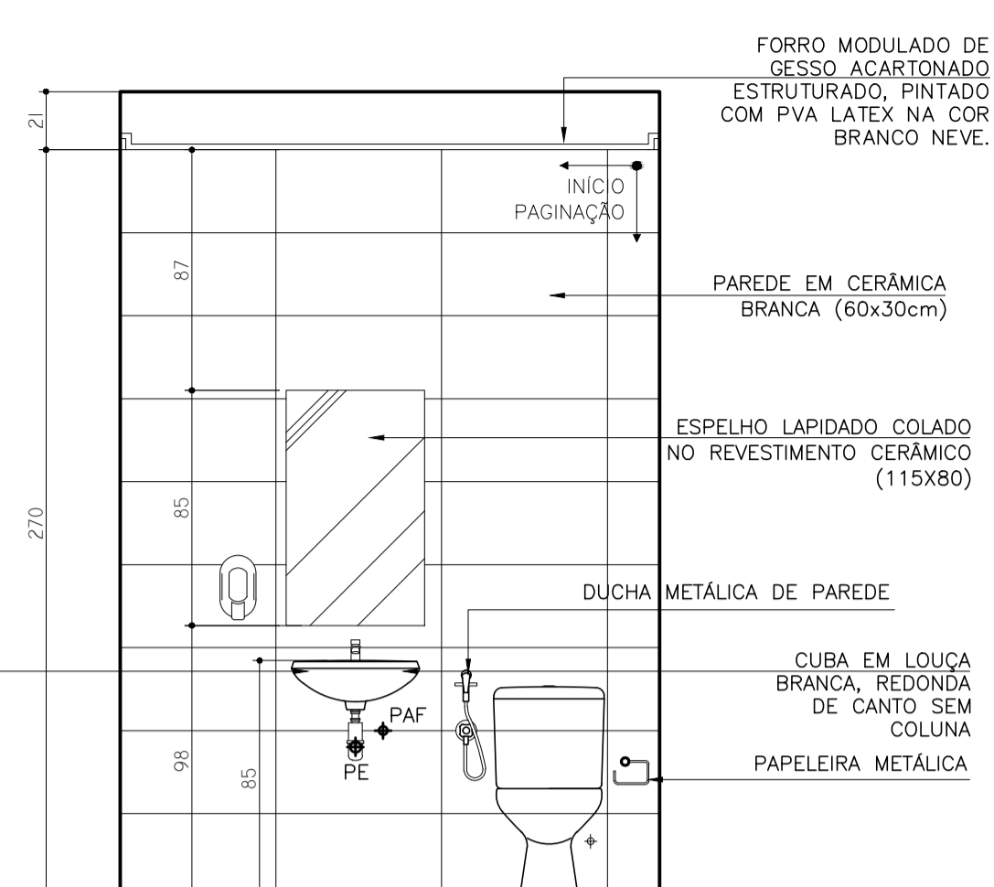
VISTA 02 LAVABO 02 ESCALA 1:25
