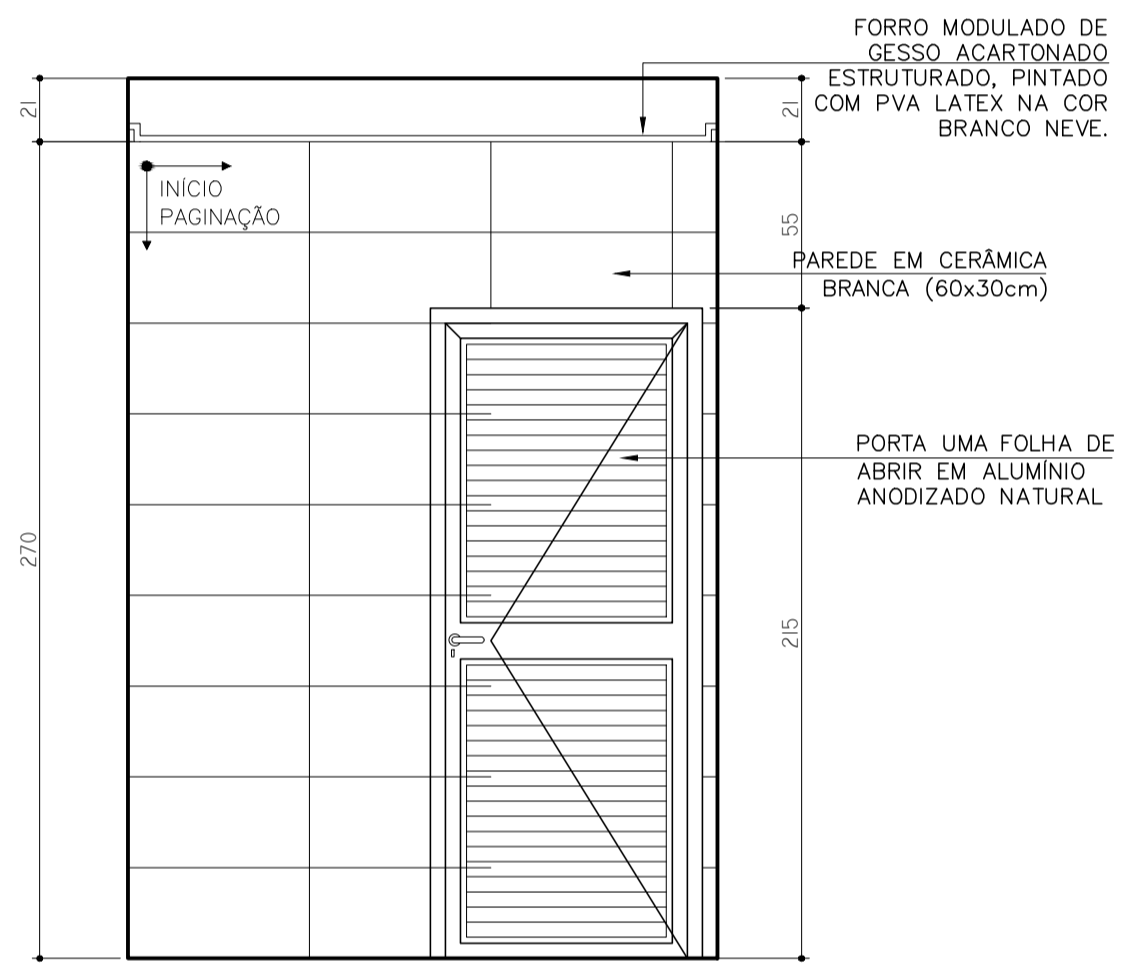
VISTA 04 LAVABO 01 ESCALA 1:25
