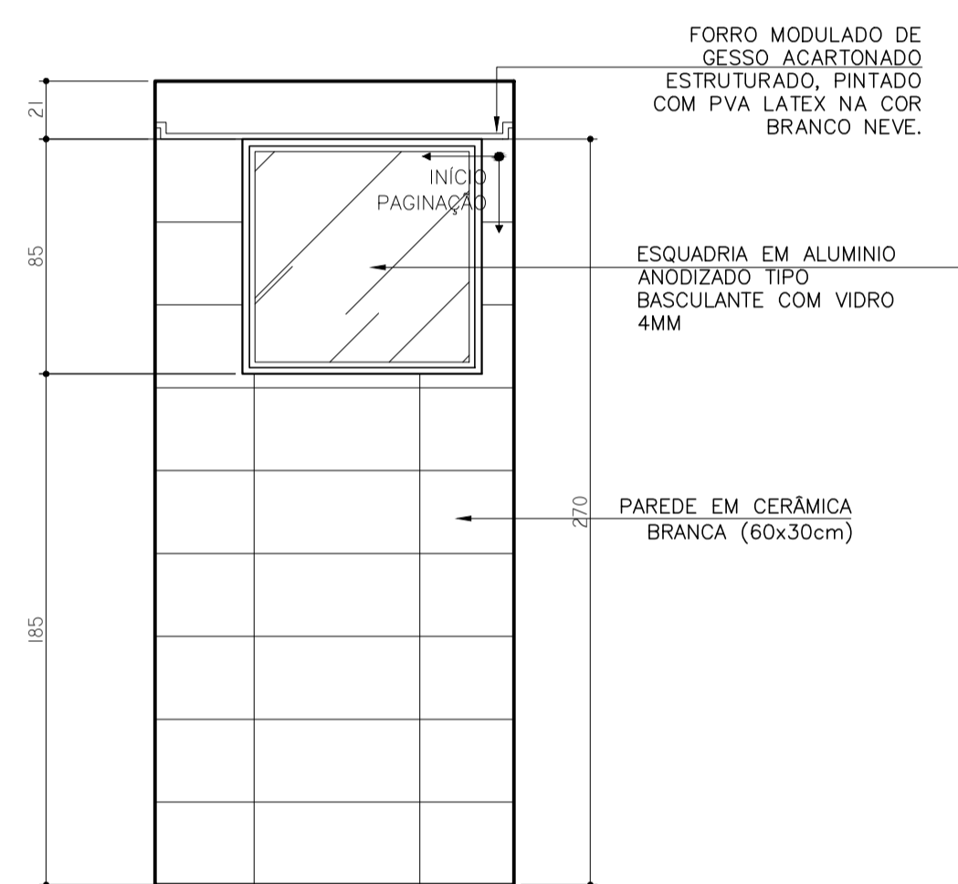
VISTA 03 LAVABO 01 ESCALA 1:25
