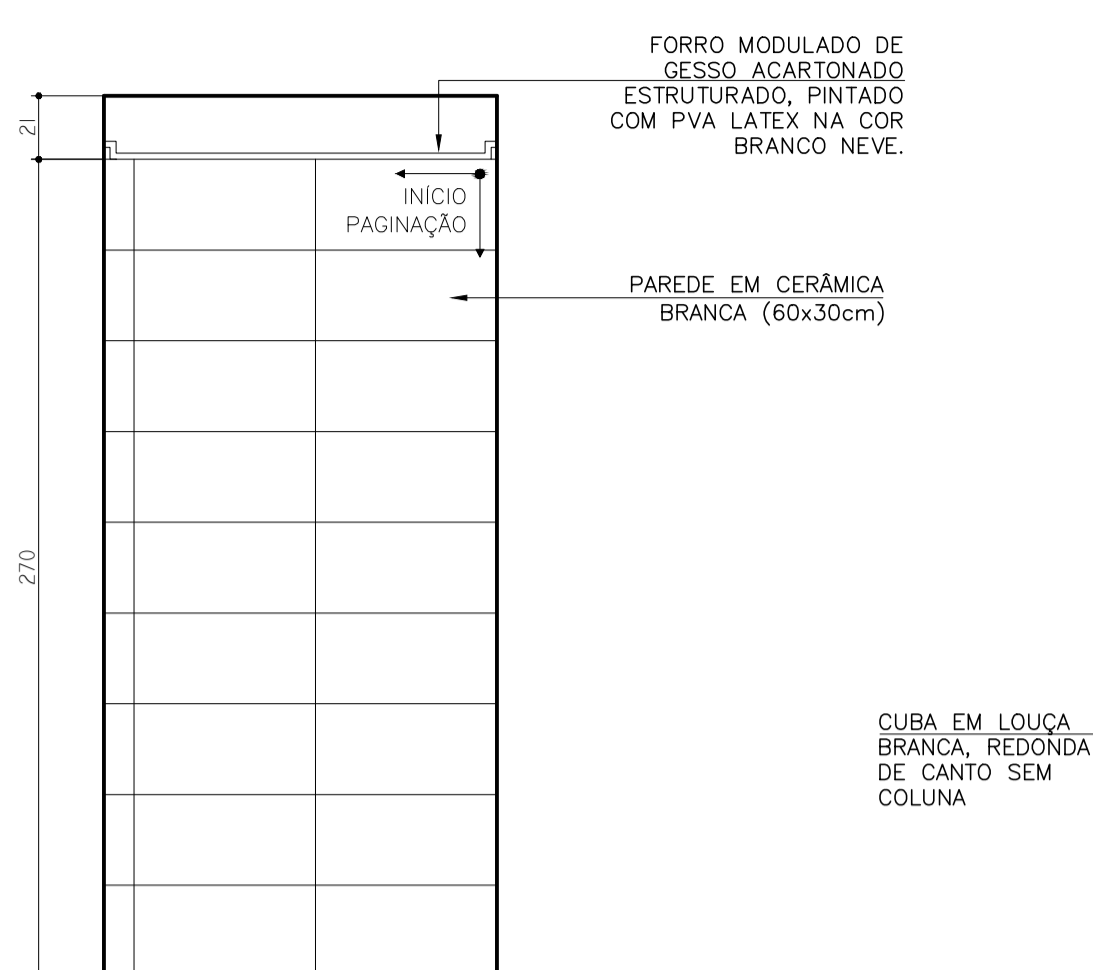
VISTA 01 LAVABO 01 ESCALA 1:25
