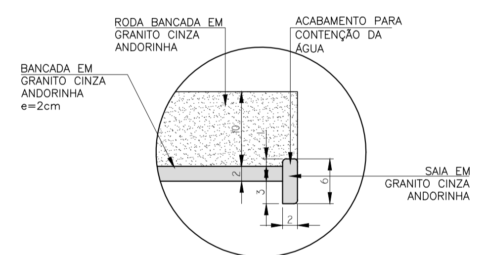
BANCADA DE GRANITO ÁREA MOLHADA esc.: 1/5
