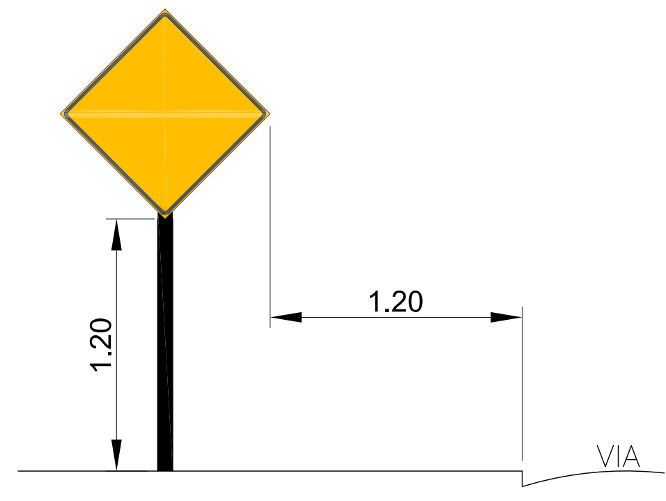
DETALHE SINALIZAÇÃO VERTICAL ESC.: 1:50
