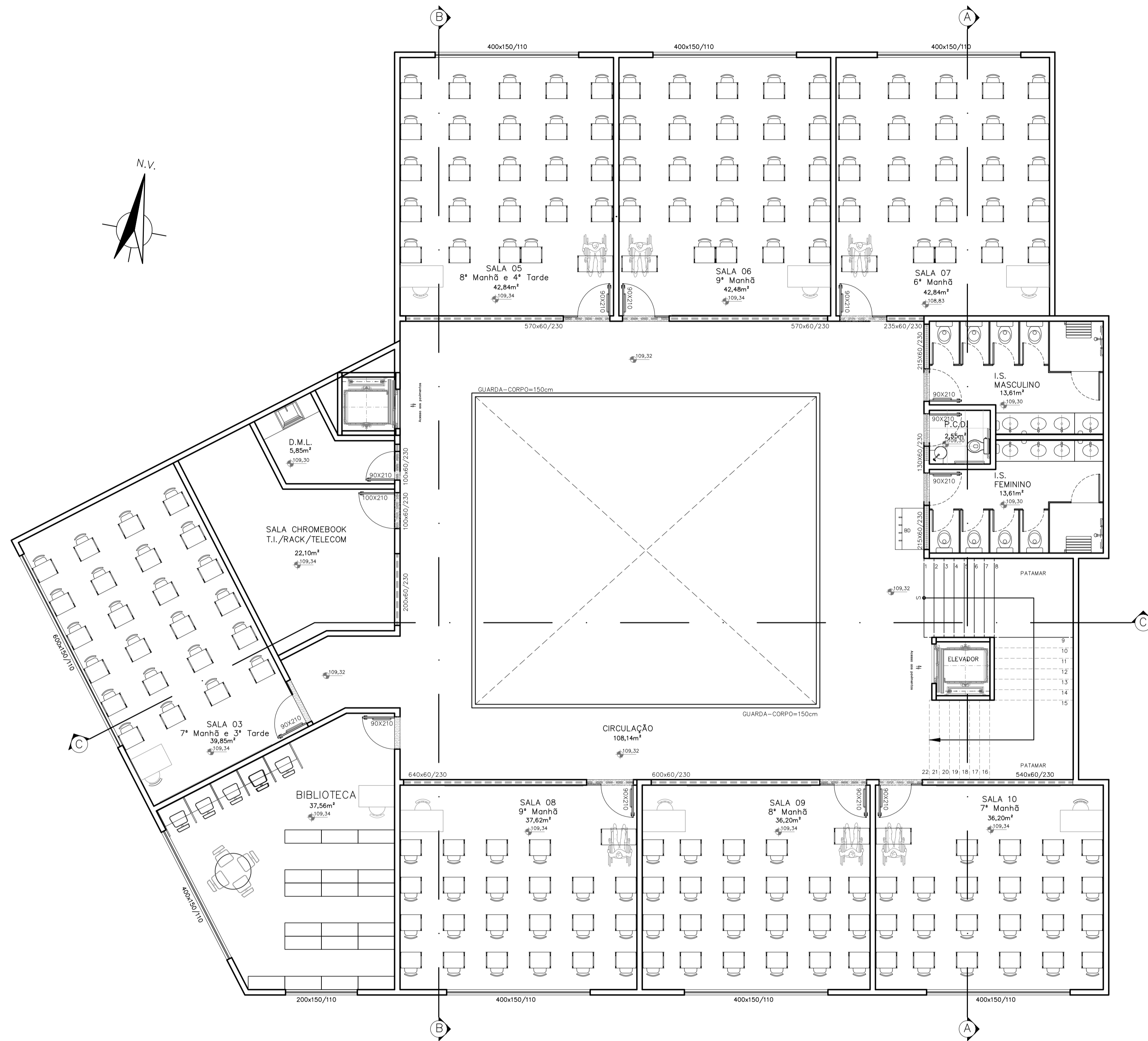
PLANTA LAYOUT 3º PAVIMENTO ESCALA 1:75
