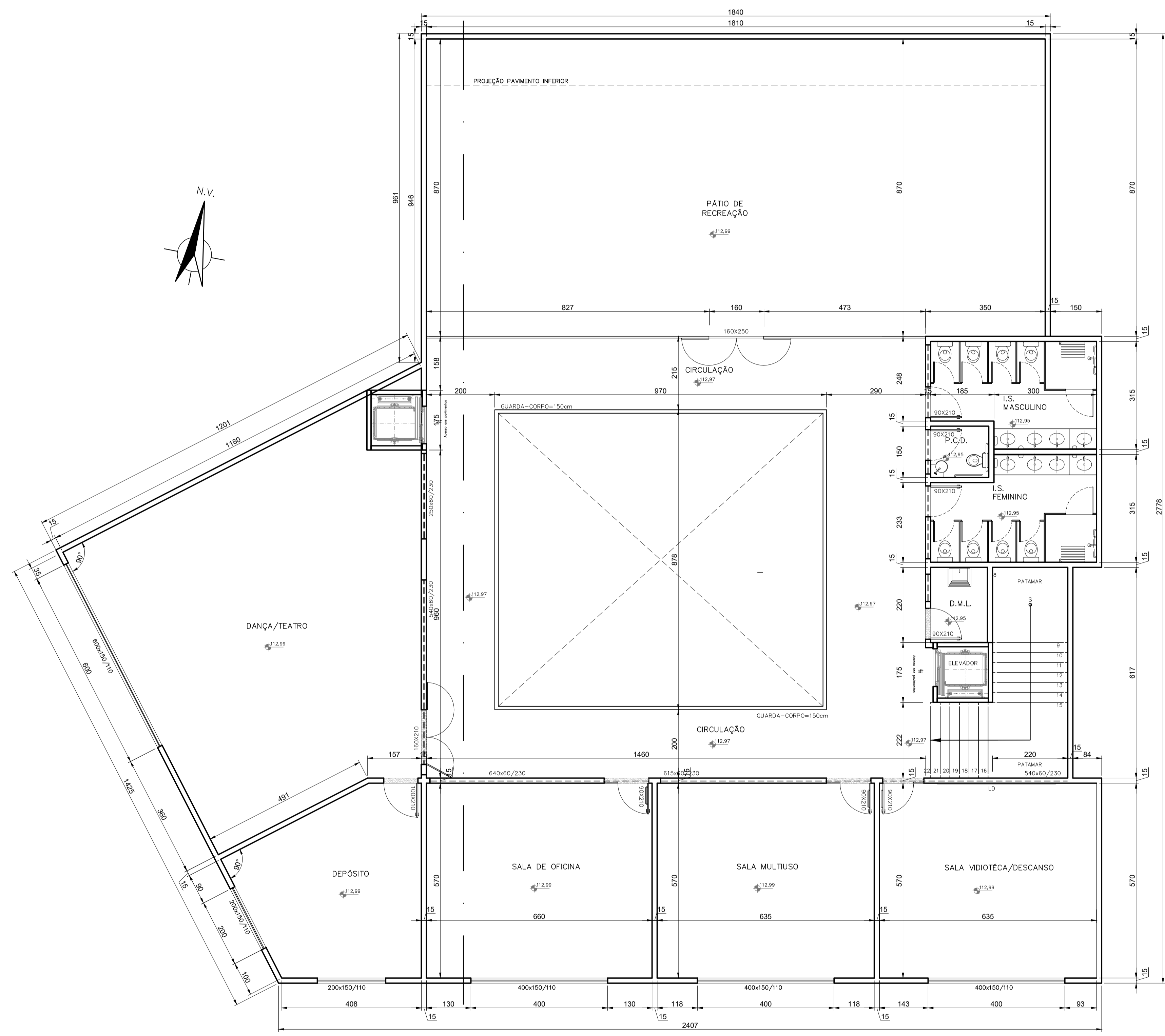
PLANTA DE DIMENSIONAMENTO 4º PAVIMENTO ESCALA 1:75
