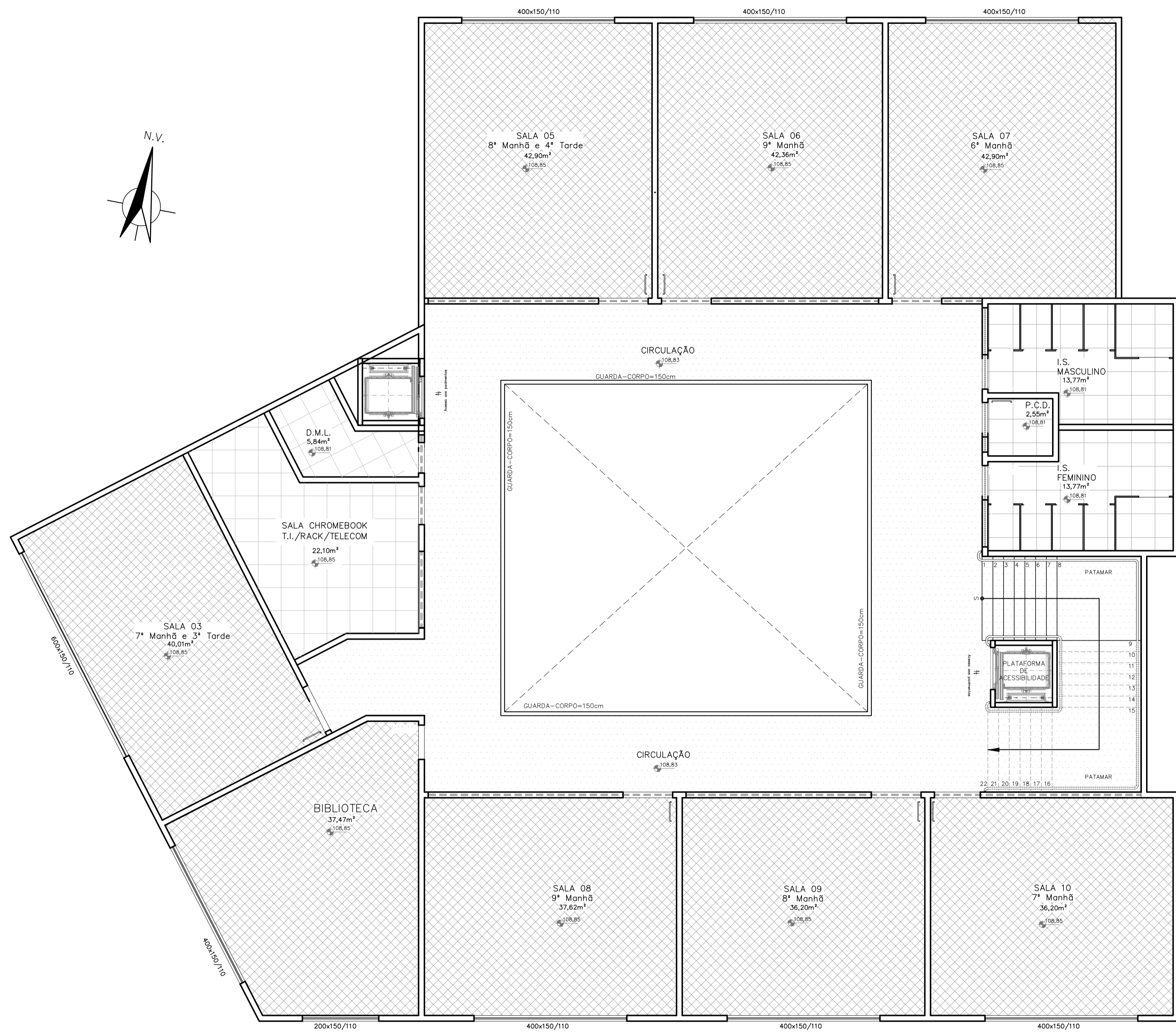
PLANTA TETO 3º PAVIMENTO ESCALA 1:75
