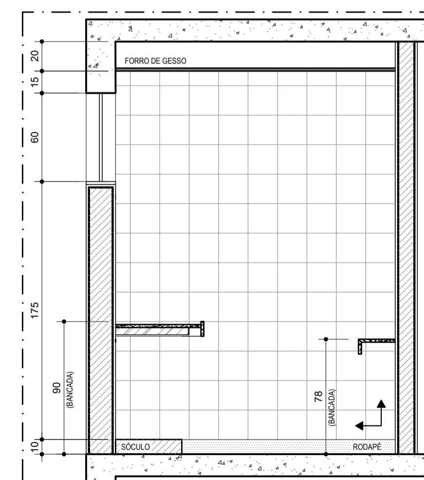
VISTA 03 DETALHE COPA ESCALA.....1/25
