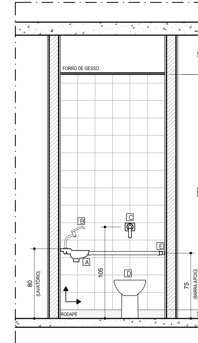
VISTA 03 DETALHE I.S. GINECOLOGIA ESCALA.....1/25
