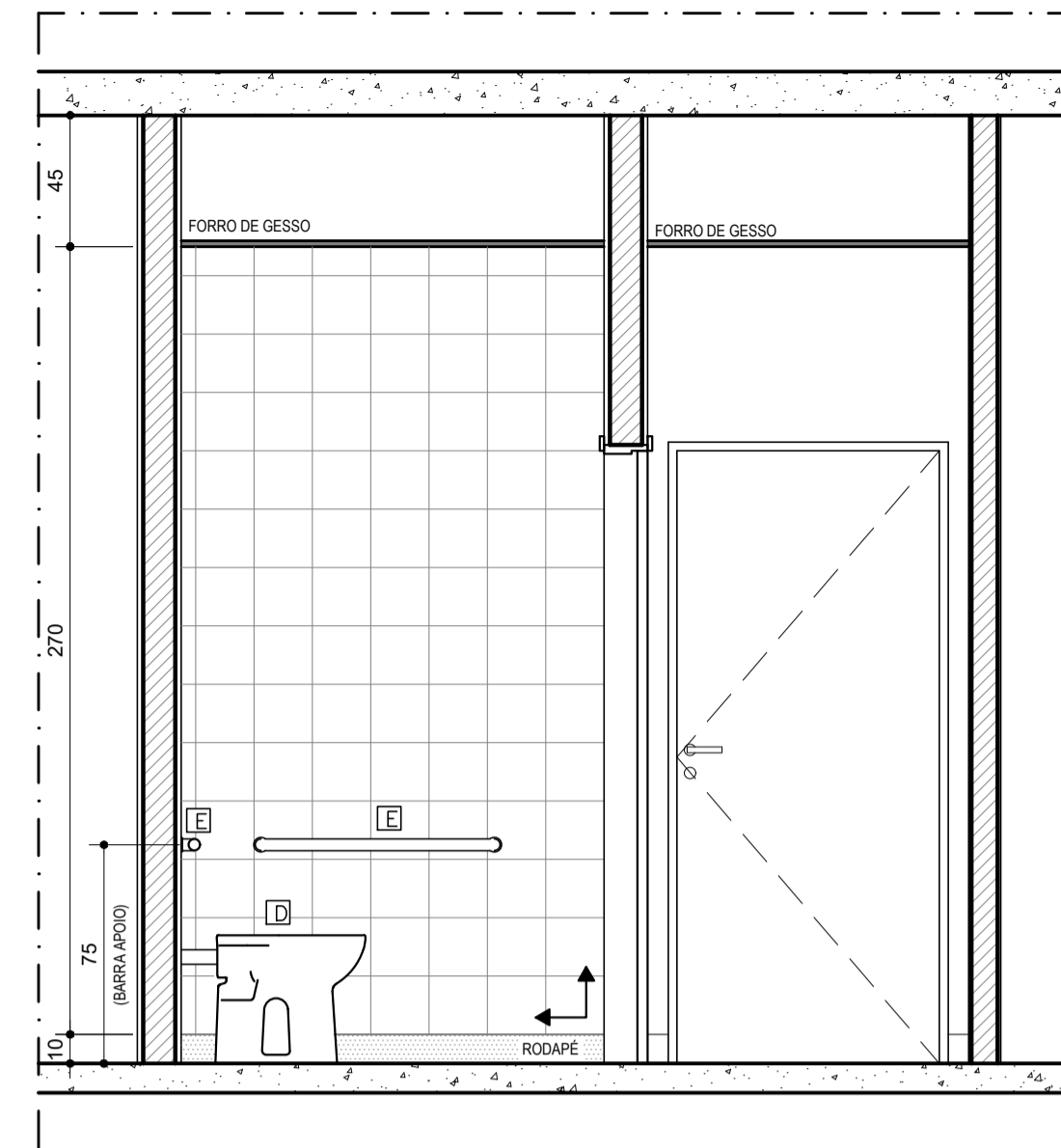
VISTA 01 DETALHE I.S. GINECOLOGIA ESCALA.....1/25
