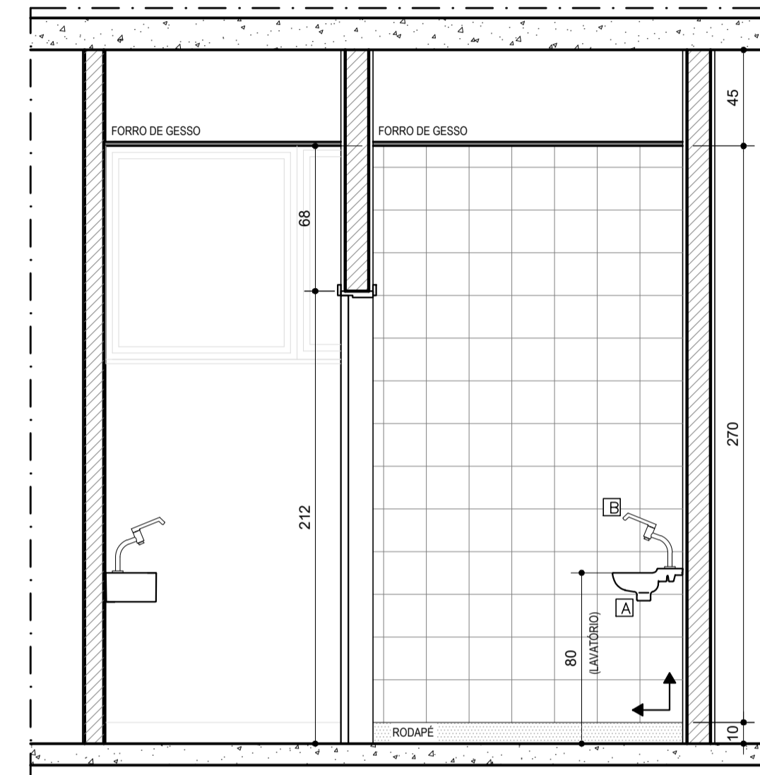
VISTA 04 DETALHE I.S. GINECOLOGIA ESCALA.....1/25
