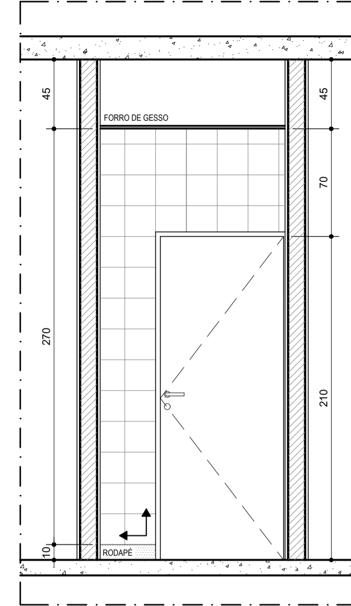
VISTA 02 DETALHE I.S. GINECOLOGIA ESCALA.....1/25
