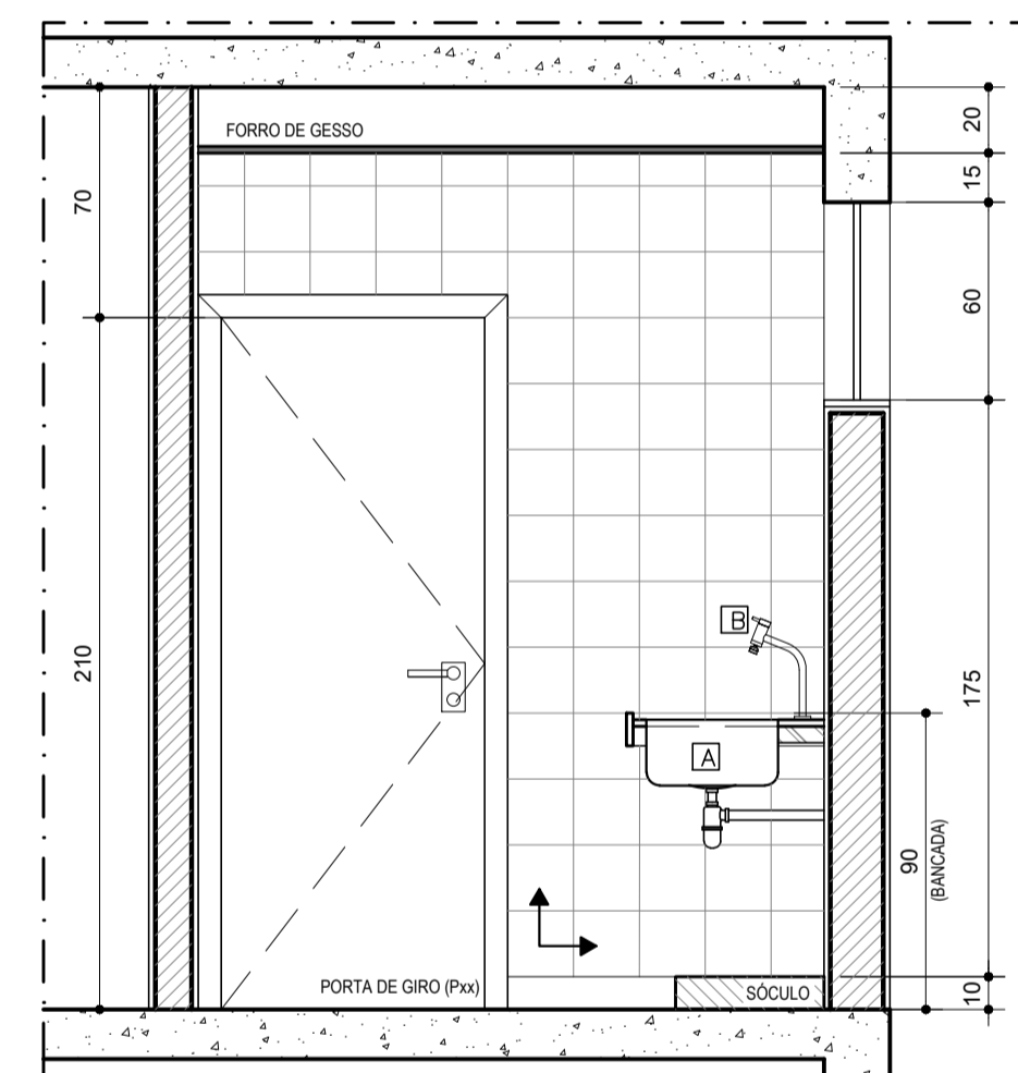
VISTA 01 DETALHE COPA ESCALA.....1/25
